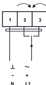
Вспомогательный переключатель
