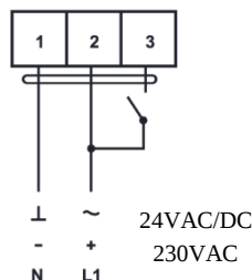
Вспомогательный переключатель
